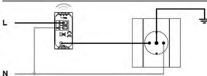
Schéma zapojenia
