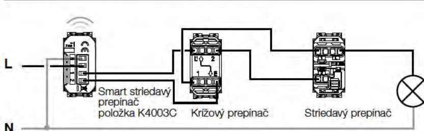
Schéma zapojenia s klasickými spínačmi č.6 a č.7
